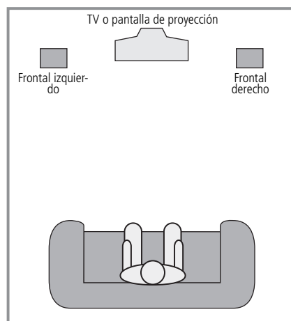
B) La distancia entre los altavoces izquierdo y derecho debe ser igual a la que hay entre las posiciones de asientos y la pantalla de visualización.
